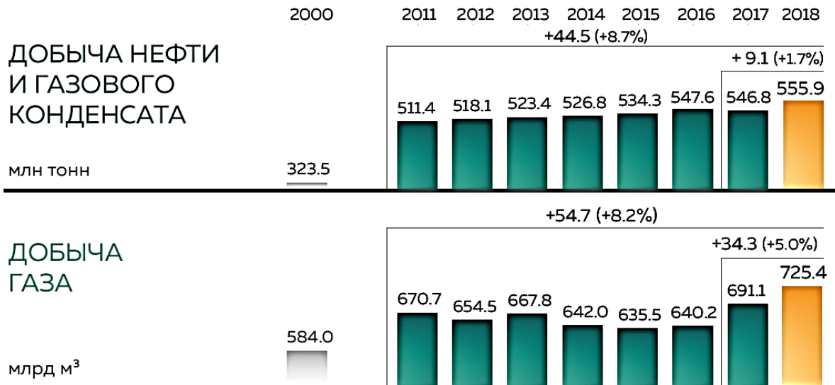
Рис. 1 - Добыча нефти и газового конденсата в России [9]
