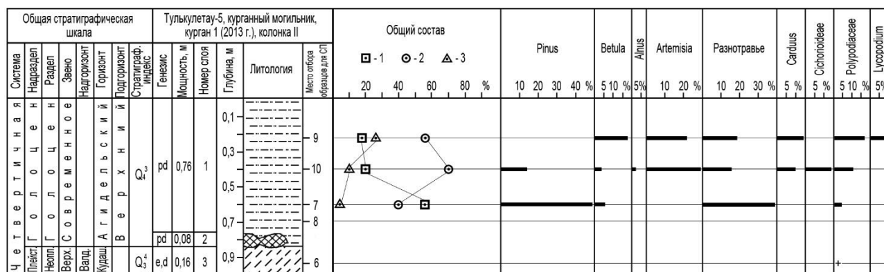
Рис. 5. Разрез плейстоценовых и голоценовых отложений курганного могильника Тулкулетау-5 и спорово-пыльцевая диаграмма (колонка II)
