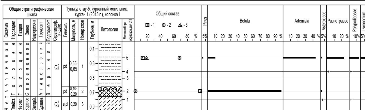
Рис 4. Разрез плейстоценовых и голоценовых отложений курганного могильника Тулкулетау-5 и спорово-пыльцевая диаграмма (колонка I).
